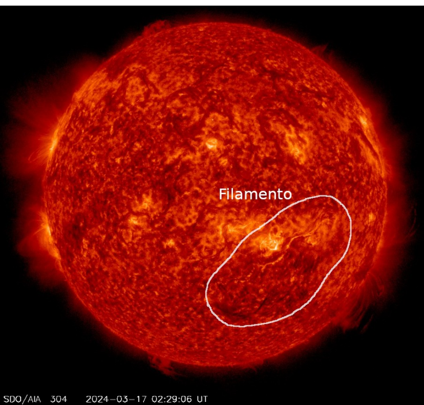
Imagen 1: https://sdo.gsfc.nasa.gov/
