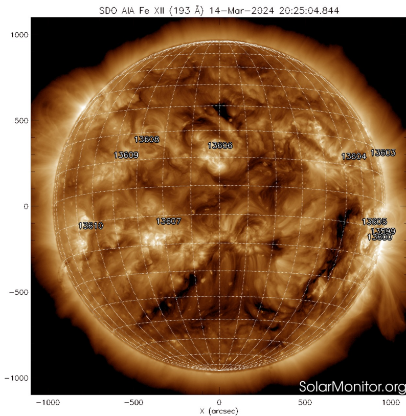
Imagen 1: https://sdo.gsfc.nasa.gov/
