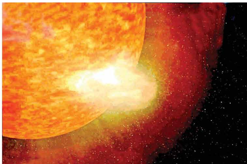
Tormentas solares.
